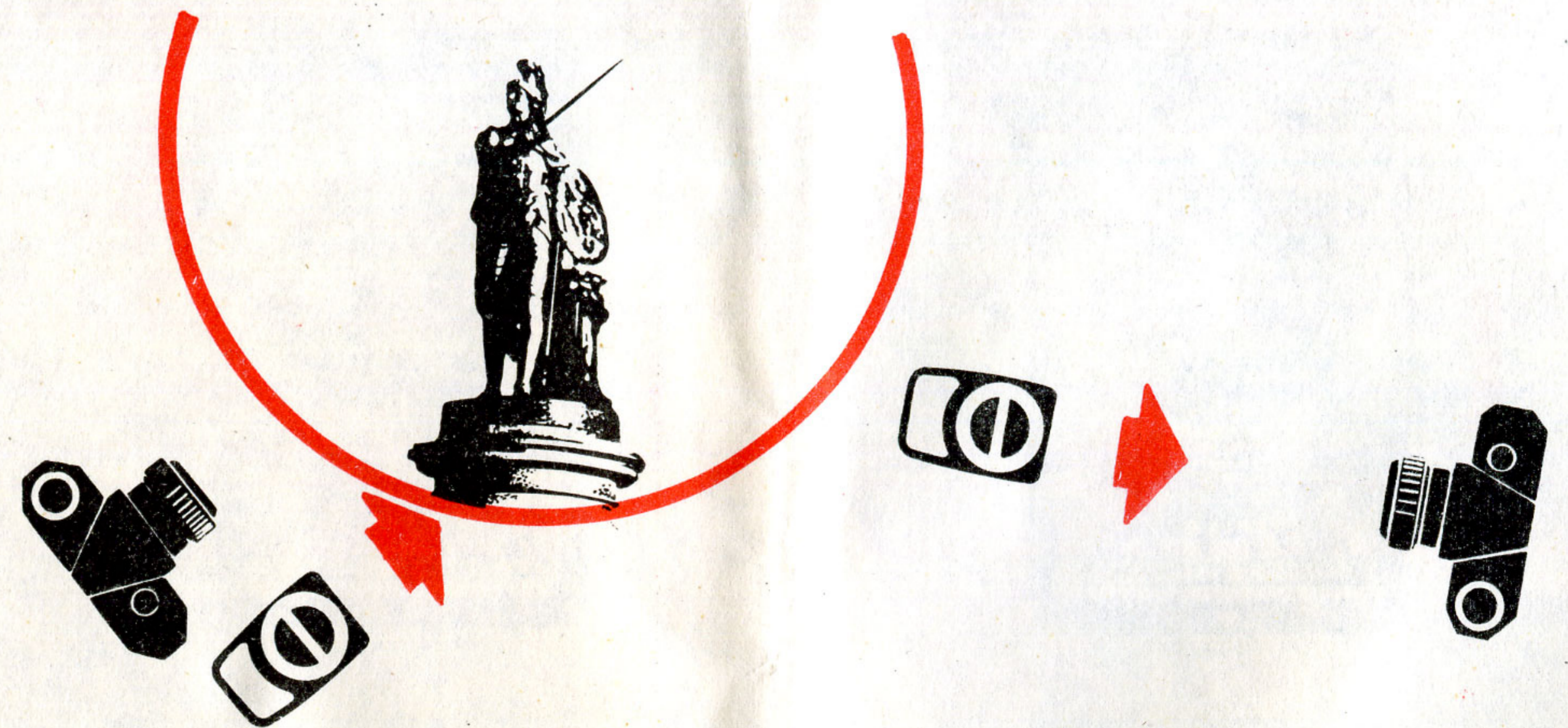
Определение выдержки или диафрагмы методом отраженного света
